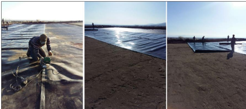
شکل (۲): عایق نمودن سطح سامانه سطوح آبخیز باران با استفاده از پوشش ژئوممبران در ایستگاه تسوج
