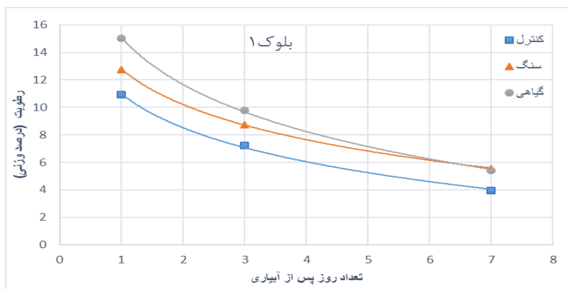
شکل ۲- تغییرات میزان رطوبت در تیمارهای پوشش خاک پوشش در روزهای مختلف بعد از آبیاری در بلوک ۱
