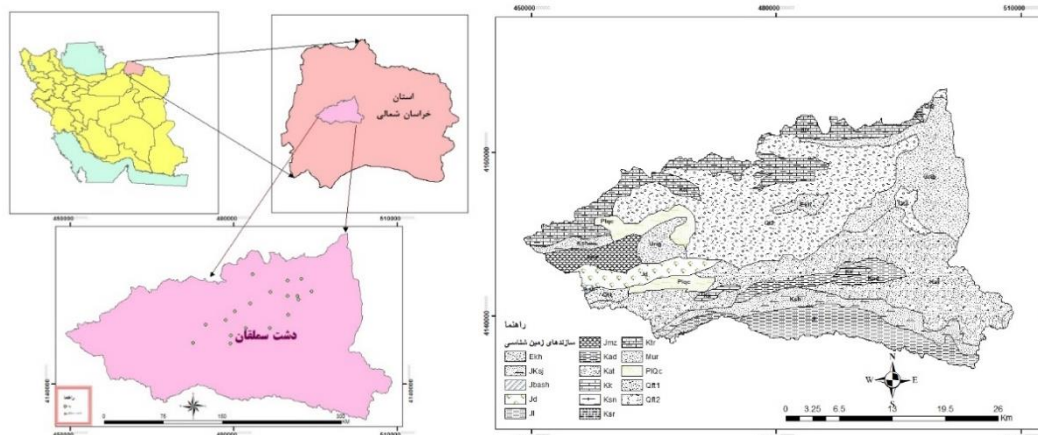
شکل ۱- موقعیت حوضه مورد مطالعه و نقشه زمین‌شناسی آن Figure 1- Location of the study watershed and its geological map
