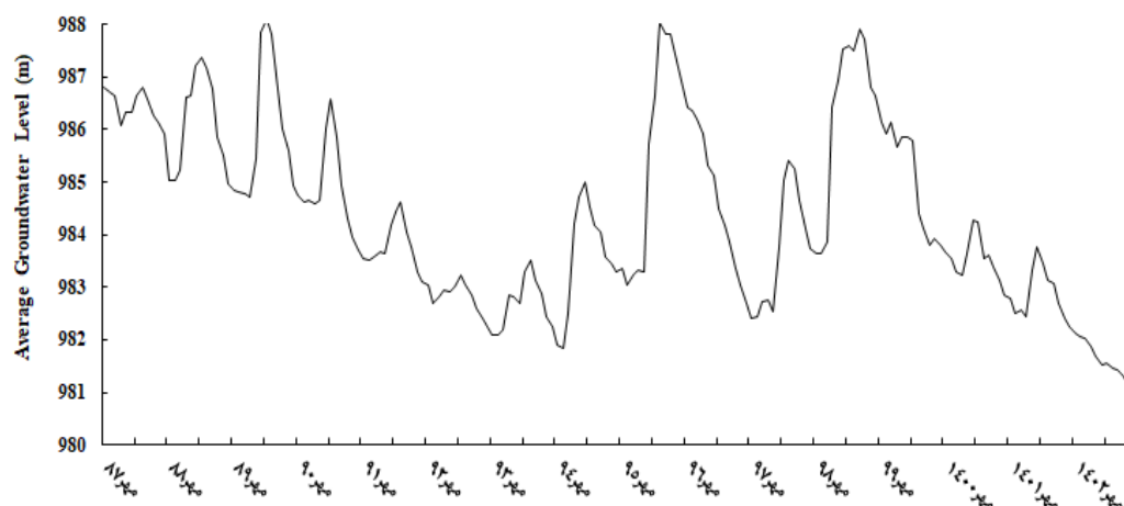
شکل ۲- هیدروگراف معرف آبخوان در منطقه مورد مطالعه
