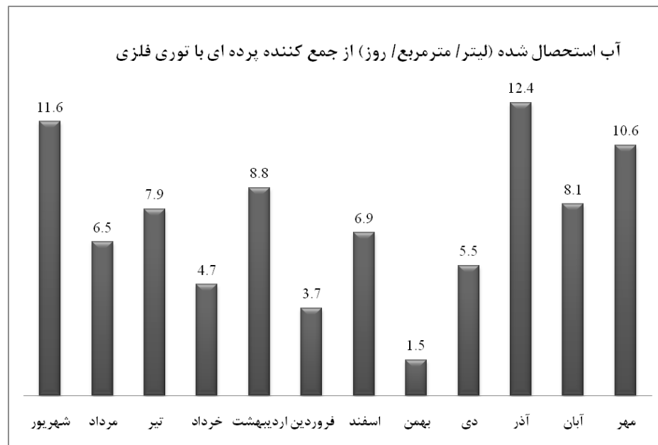
شکل ۷- نمودار میانگین ماهانه آب استحصال‌ی از جمع‌کننده پرده‌ای با توری فلزی (لیتر / مترمربع / روز)
