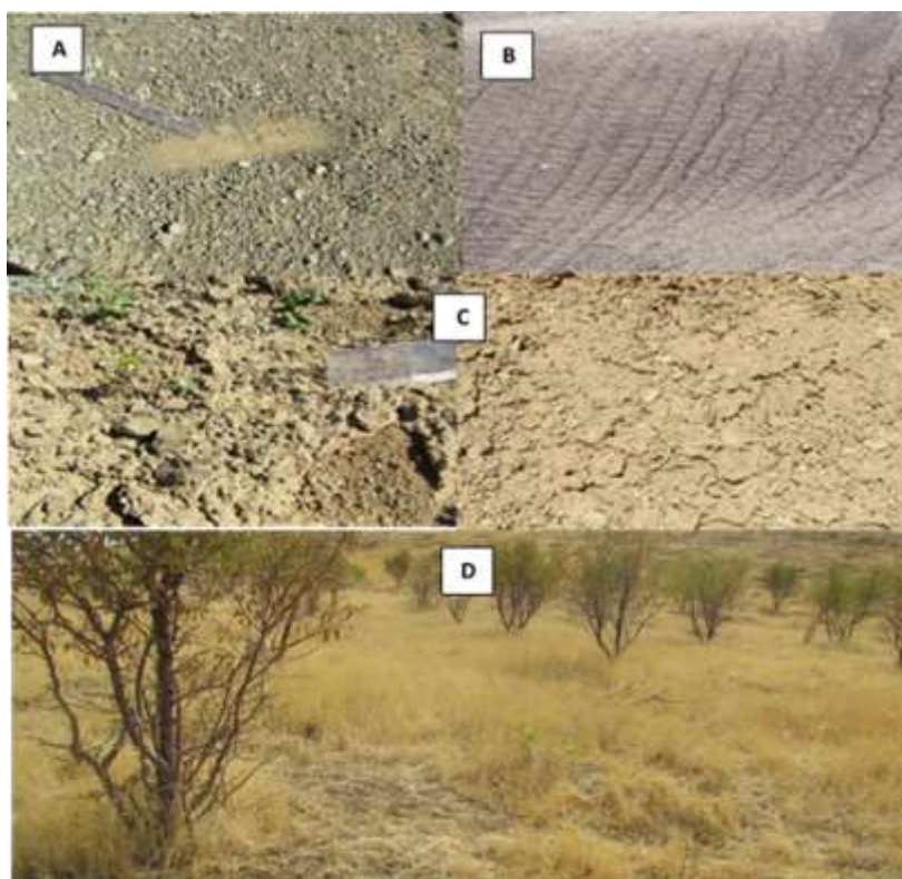
شکل (۵): اشکال ظاهری تخریب خاک (آرمور A، فرسایش شیاری B و کراست سطحی C) در دیمزارهای شیب‌دار شاهد و مه‌آنها در عرصه بادام کاری D
