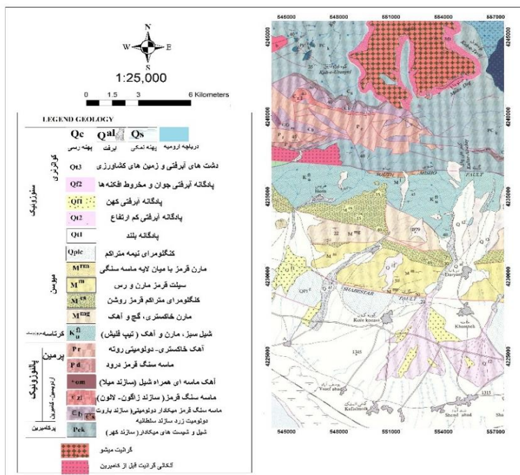
شکل (۵): نقشه زمین‌شناسی حوزه آبخیز (برگرفته از نقشه زمین‌شناسی ۱:۰۰۰۰۰ موند)
