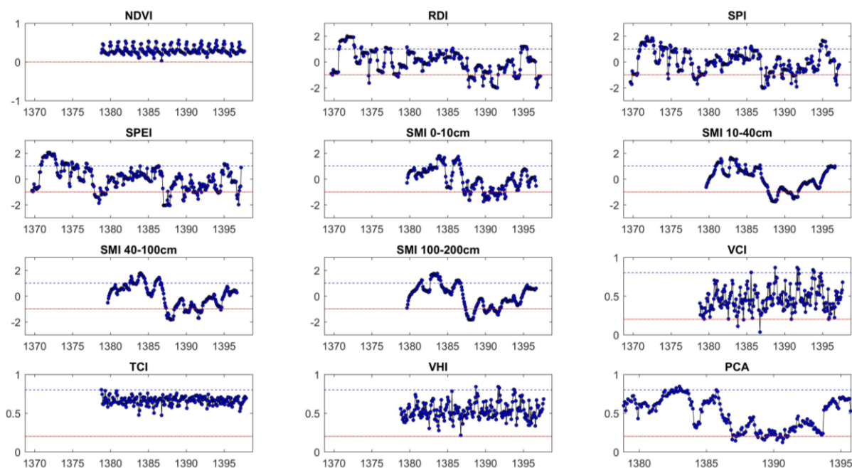
شکل (۴): سری زمانی شاخص‌های مختلف خشکسالی در مقیاس زمانی ۱۲ ماهه (SPEI, RDI, NDVI, SMI, VCI, TCI, VHI, PCA)
