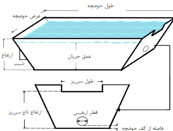
شکل ۴- طرح شماتیک حوضچه تاخیری ذوزنقه‌ای با خروجی ارفیس دایره‌ای و سرریز مستطیلی Figure 4- Schematic design of trapezoidal delay catchment with circular orifice outlet and rectangular overflow
