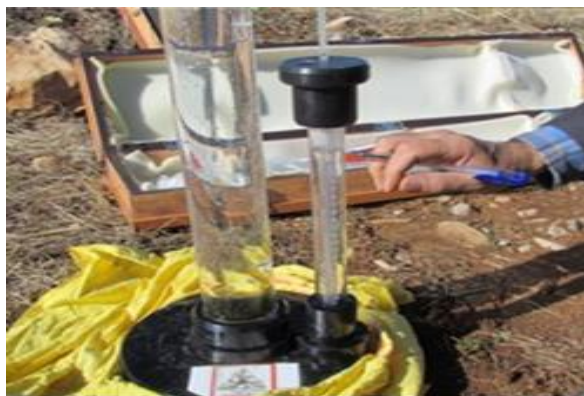
شکل ۲- روش اندازه‌گیری نفوذپذیری خاک به کمک دستگاه نفوذسنج صفحه‌ای
