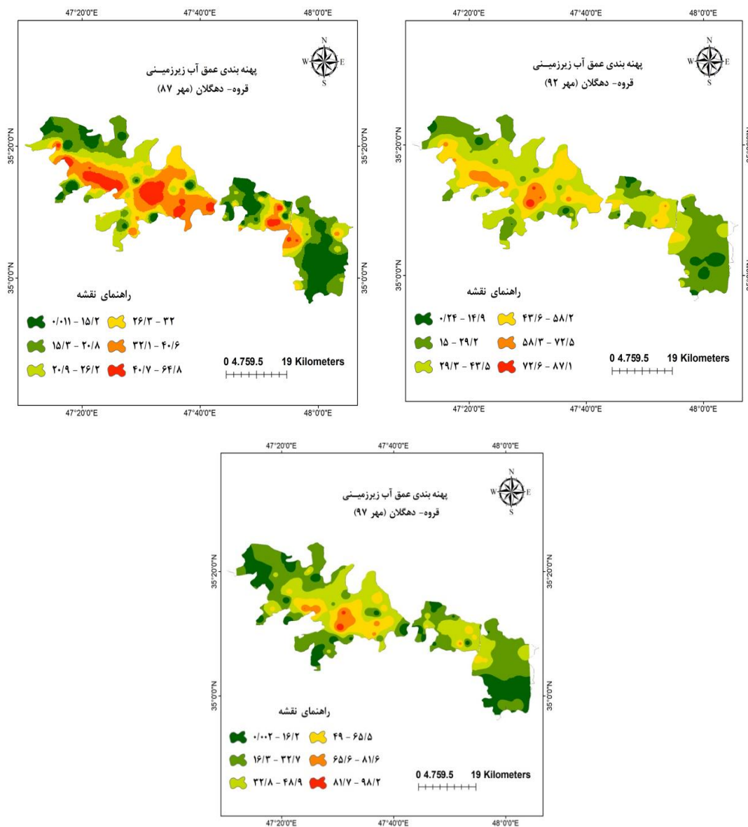
شکل ۲- پهنه‌بندی عمق آب زیرزمینی آبخوان قروه- دهگلان در سال‌های ۱۳۸۷، ۱۳۹۲ و ۱۳۹۷ Figure 2- Zoning of the groundwater depth of Gorveh-Dehghan aquifer in the years 2008, 2012, and 2018
