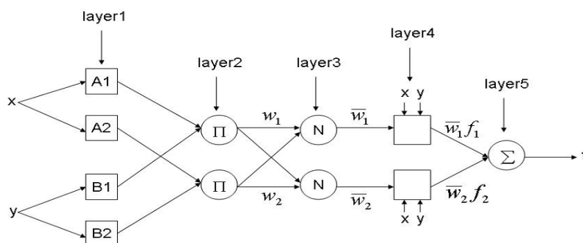
شکل ۴- ساختار یک شبکه ANFIS با دو ورودی (Azimi et al., 2018) Figure 4- Structure of ANFIS model with two inputs (Azimi et al., 2018)
