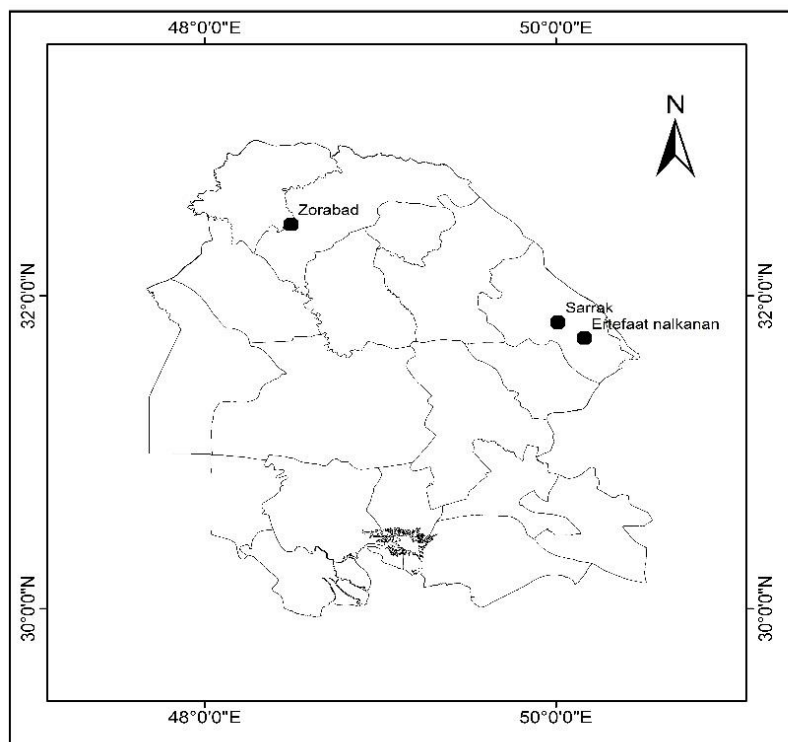
شکل ۲- پراکندگی ایستگاه‌های ناهمگن بر اساس آزمون بیشاند برای استان خوزستان Figure 2- The distribution of heterogeneous stations based on Buishand test for Khuzestan province
