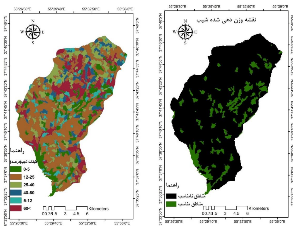
شکل ۶- نقشه طبقه‌بندی کلاس‌های شیب حوزه آبریز قویجق
