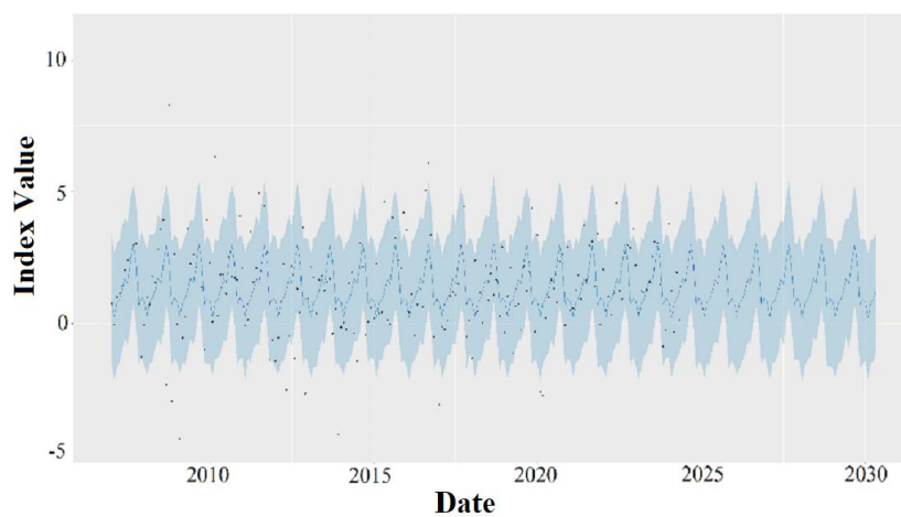
شکل ۱۰- نمودار پیش‌بینی مدل فیسبوک پروفیت برای شاخص VWR Figure 10- Forecast chart of the facebook prophet model for the VWR index
