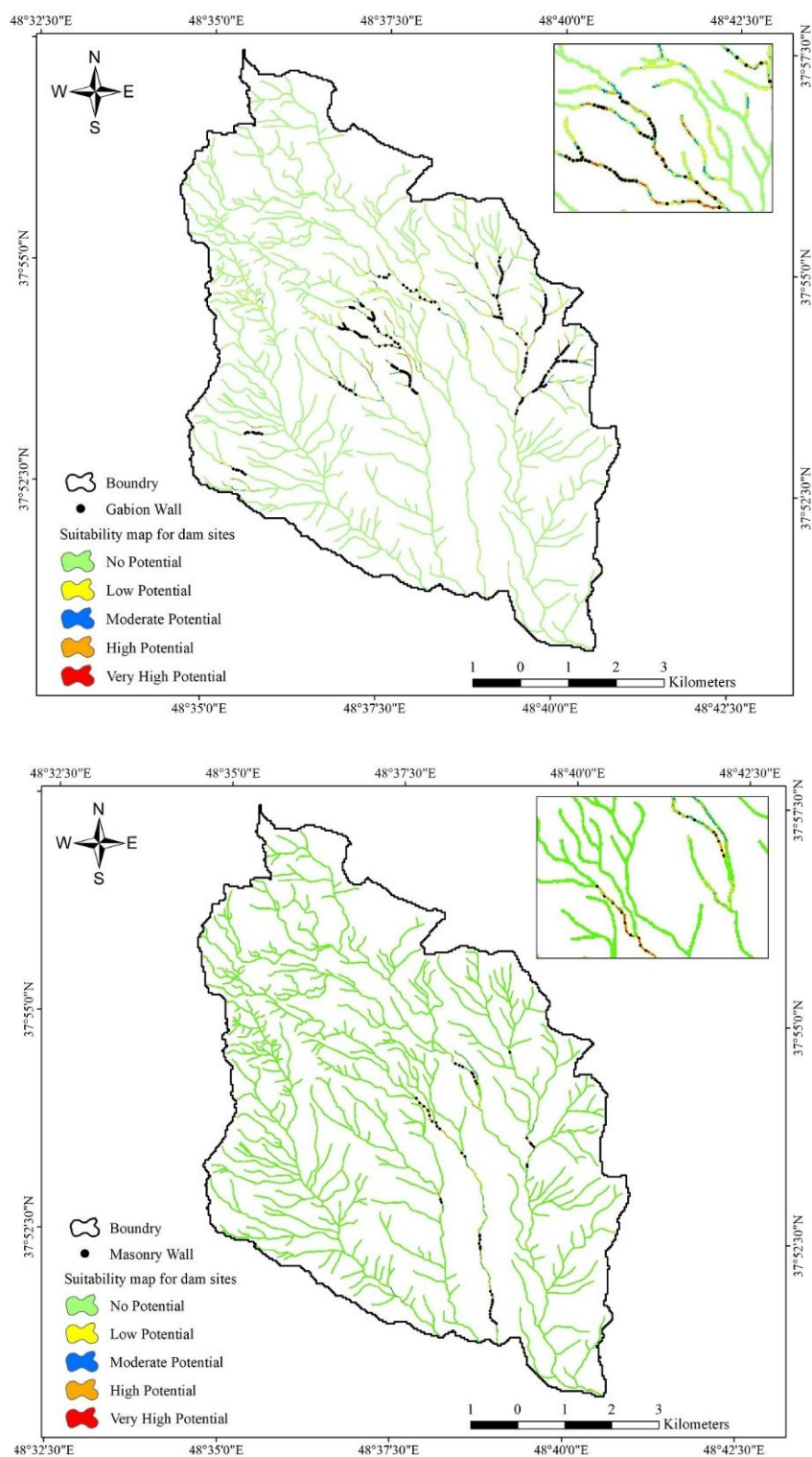
شکل ۷- نقشه نهایی پتانسیل احداث سازه‌های گابیونی (تصویر بالا) و سنگی ملاتی (تصویر پایین) در حوزه آبخیز آق‌اولر Figure 7- Final potential map for the construction of gabion (top image) and masonry wall (bottom image) structures in the Aghevlar watershed
